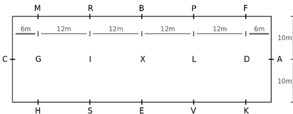
СХЕМА МАНЕЖА 20 x 60 м
