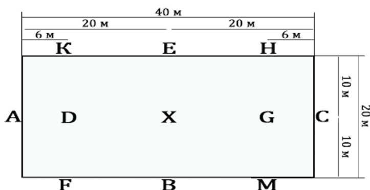
СХЕМА МАНЕЖА 20 x 40 м
